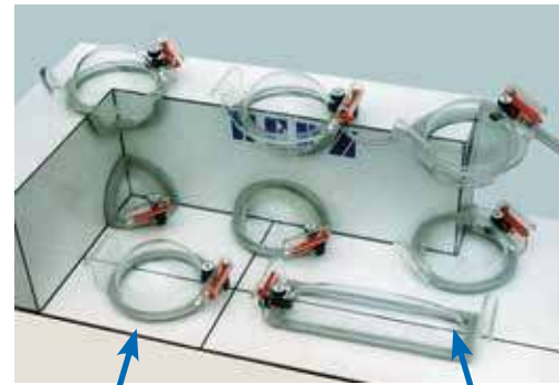
Prüfglocken-Set rund
